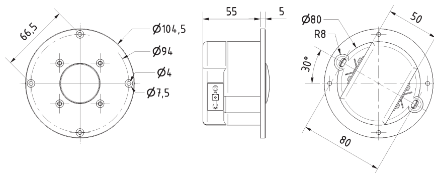
KE 25 SC - 8 Ohm
