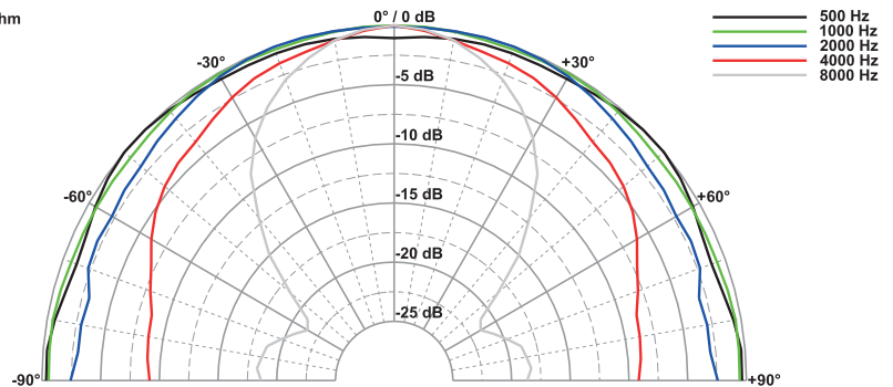
B 80 – 8 Ohm 17.09.2012
