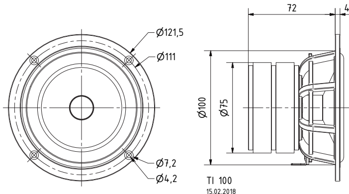
TI 100 - 8 Ohm
